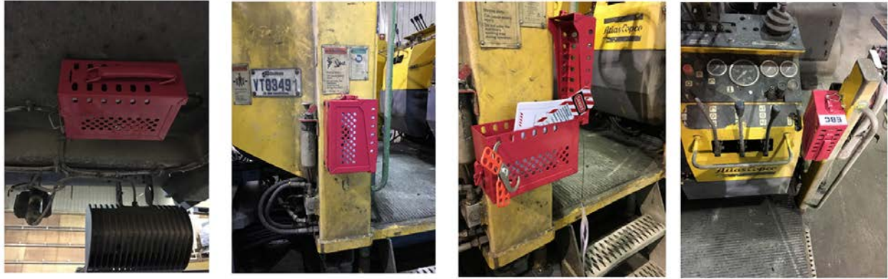
Photo de la boîte de cadenassage (Gracieuseté EBC Mines)
